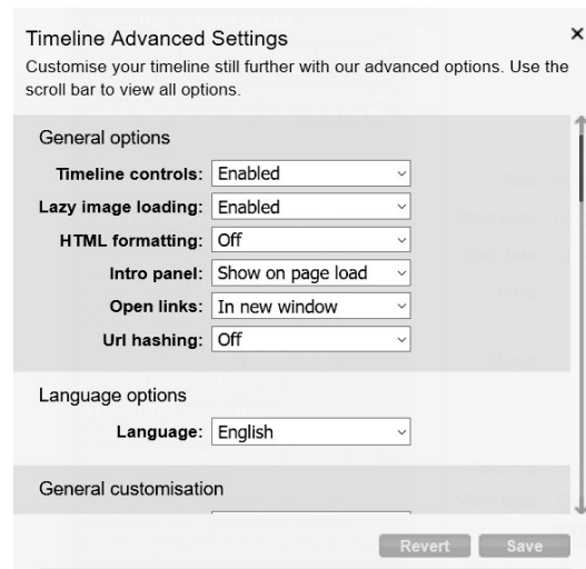
Рис. 5. Окно дополнительных параметров в сервисе Tiki-Toki
