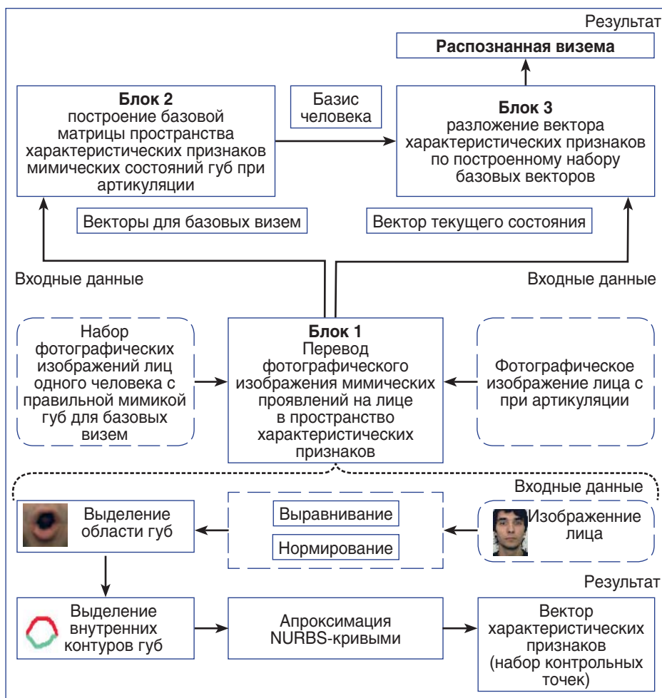
Рис. 3. Схема чтения по губам слов на украинском языке
