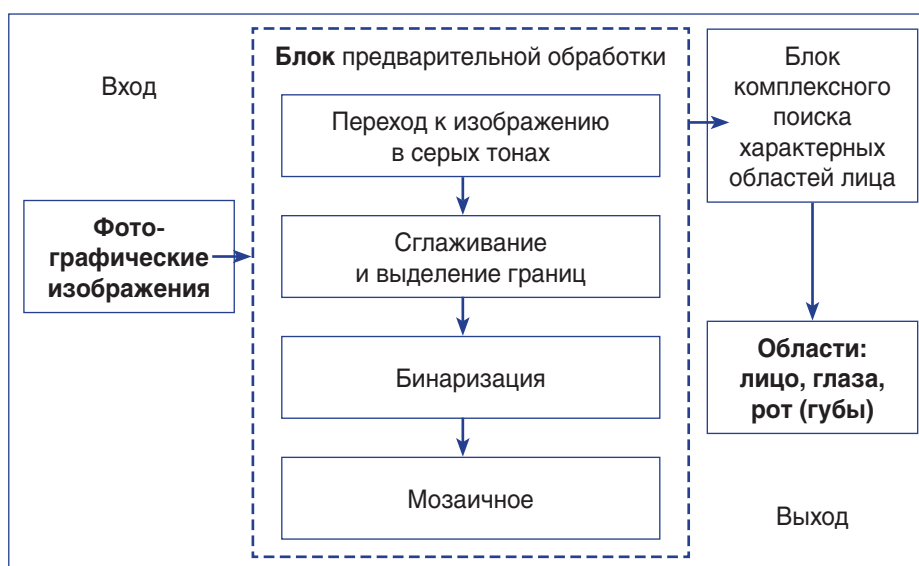
Рис.1. Общая схема алгоритма комплексного поиска областей лица человека на фотографическом изображении
