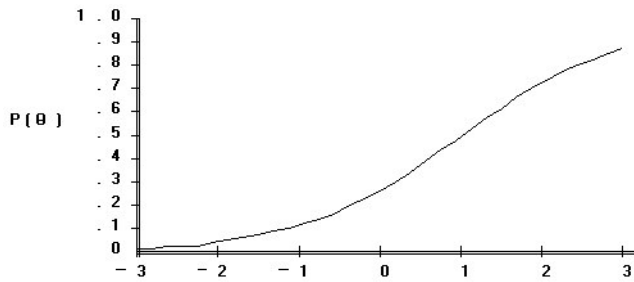
Рис. 3. График функции P(\theta) при уровне трудности задания \beta_j = 1
