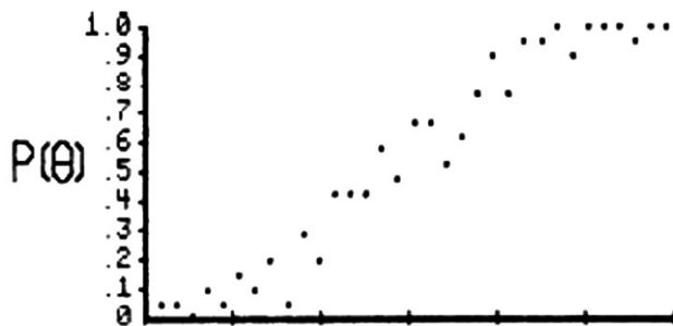
Рис. 4. Эмпирически полученные значения долей правильных ответов на задание теста в каждой балльной группе испытуемых
