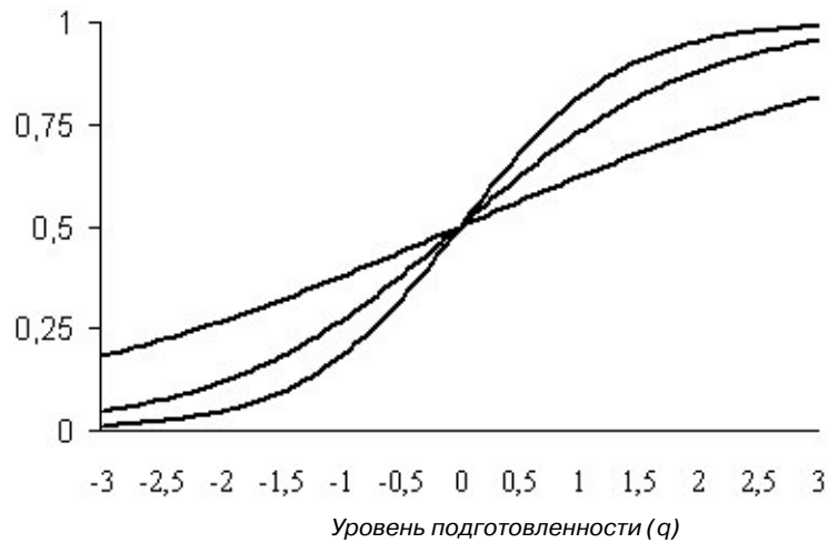
Рис. 1. Вероятностные функции (графические образы) заданий одинакового уровня трудности, отличающиеся значениями параметра дифференцирующей способности a_j : a_1 = 1,5 ; a_2 = 1,0 ; a_3 = 0,5 .
