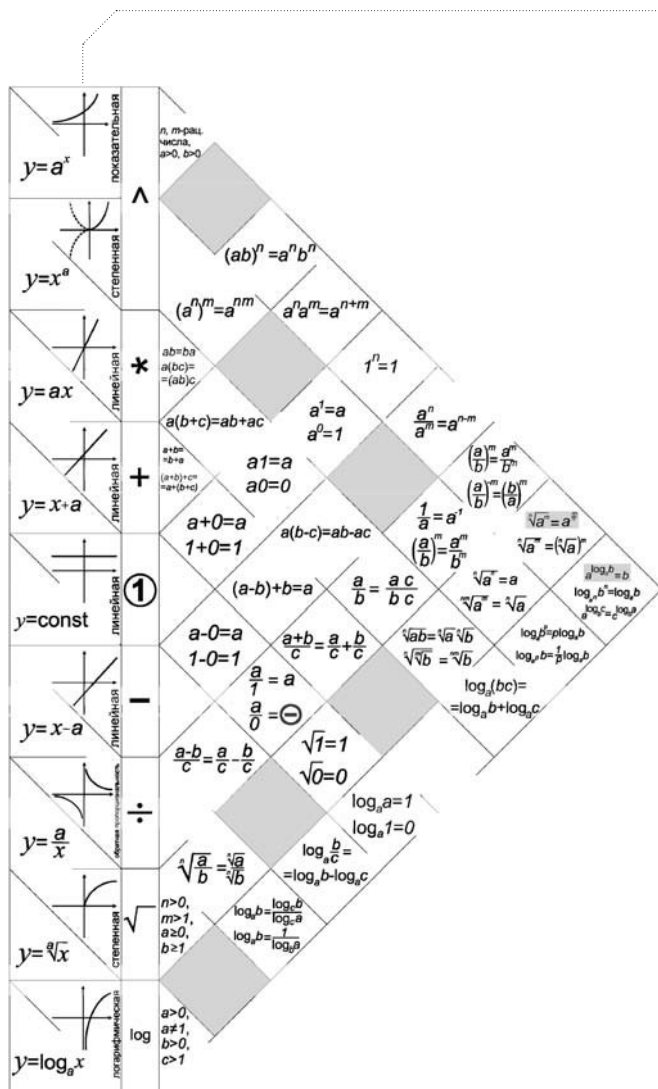
Рис. 2. Полная линейно-матричная модель «Математические действия и их свойства, функции и их графики»
