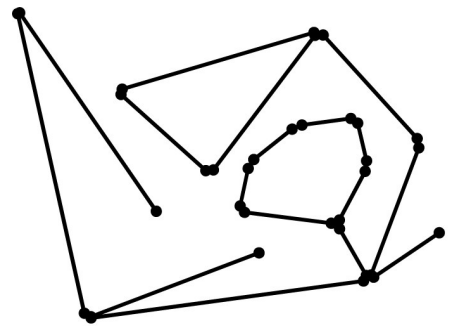
Связный граф
