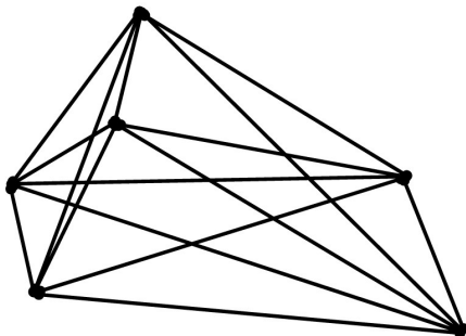
Полный граф
