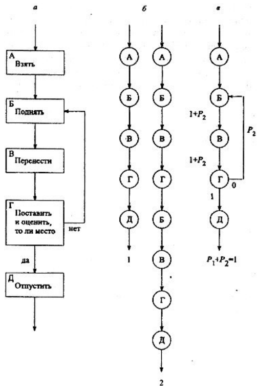
Рис. 1. Графы алгоритмов:
