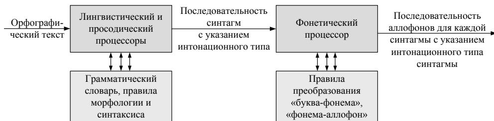
Рис. 2. Структура модуля обработки текста
